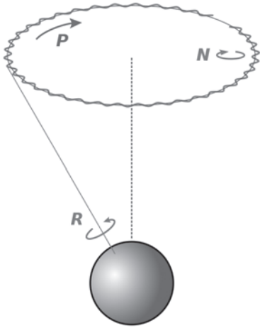
ന്യൂട്ടേഷൻ (Nutation)
